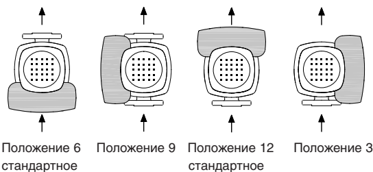
Рис. 27 Положение клеммной коробки
