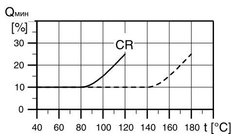
Рис. 29 Минимальная подача
