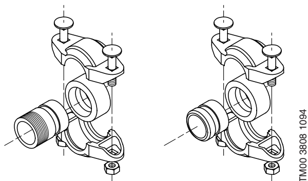
Рис. 36 Муфта PJE
