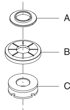
Рис. 7 Стопорное кольцо
