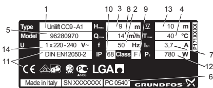
Рис. 2 Пример фирменной таблички для модели насоса Unilift CC 9
