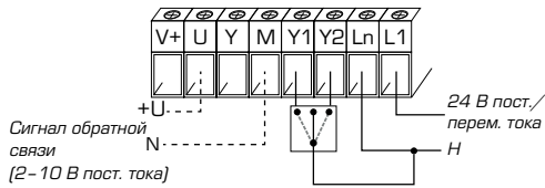
3-точечный режим управления (приемник)
