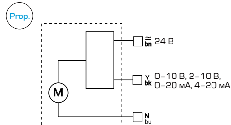
Серия ARA659 + Серия 90P
